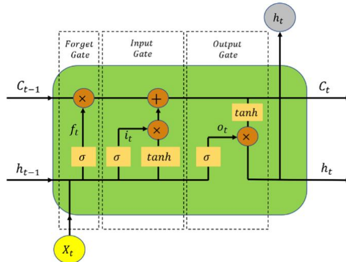
Gambar 2 Arsitektur LSTM
